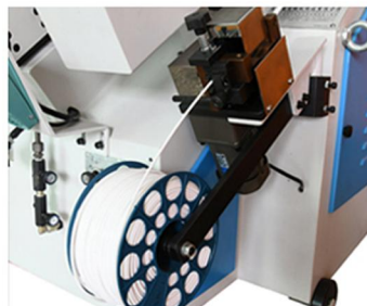
自動上膠系統 Automatic Cementing
