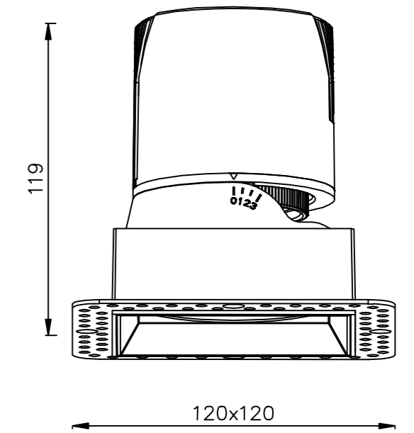
开孔: 95x95
