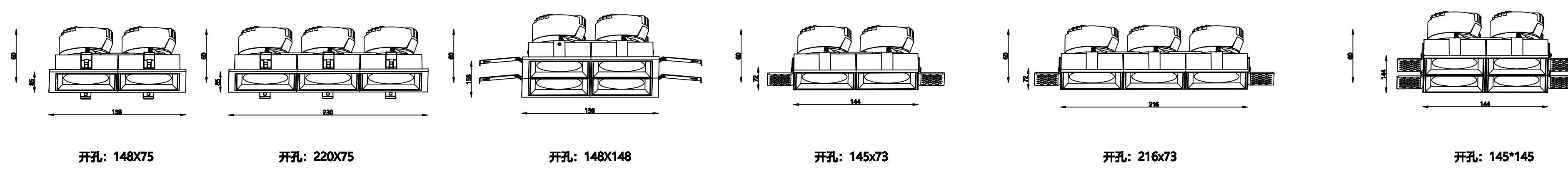
开孔: 148x75 开孔: 220x75 开孔: 148x148 开孔: 145x73 开孔: 216x73 开孔: 145x145
