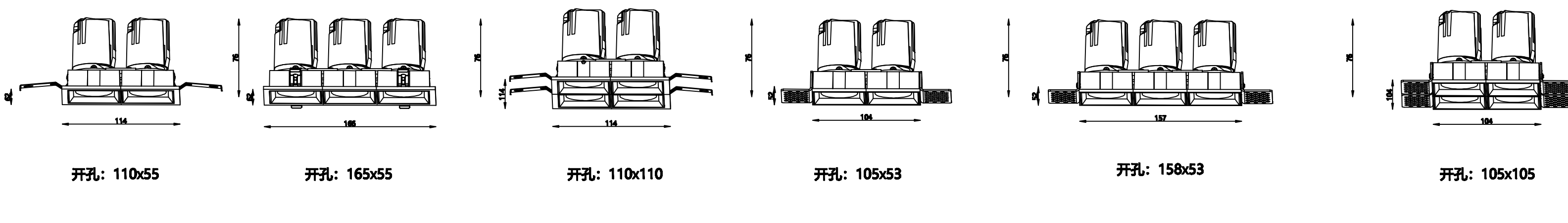
开孔: 110x55 开孔: 165x55 开孔: 110x110 开孔: 105x53 开孔: 158x53 开孔: 105x105
