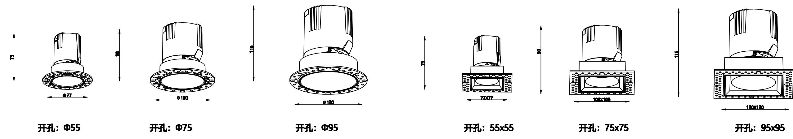
开孔: \phi 55 开孔: \phi 75 开孔: \phi 95 开孔: 55x55 开孔: 75x75 开孔: 95x95
