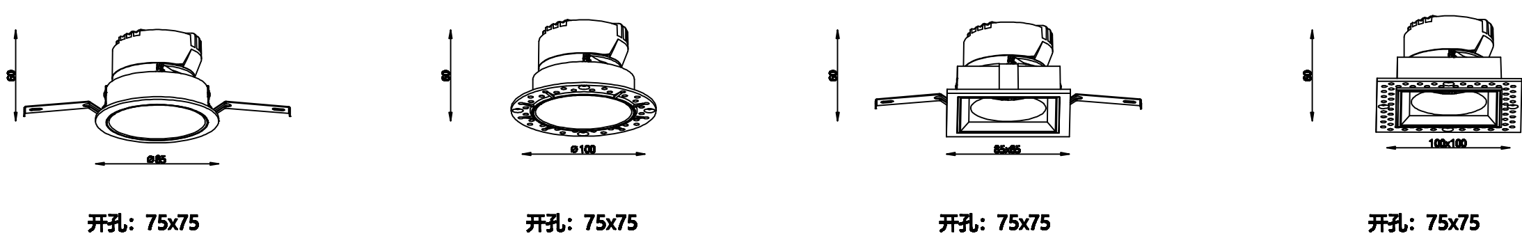
开孔: 75x75 开孔: 75x75 开孔: 75x75 开孔: 75x75
