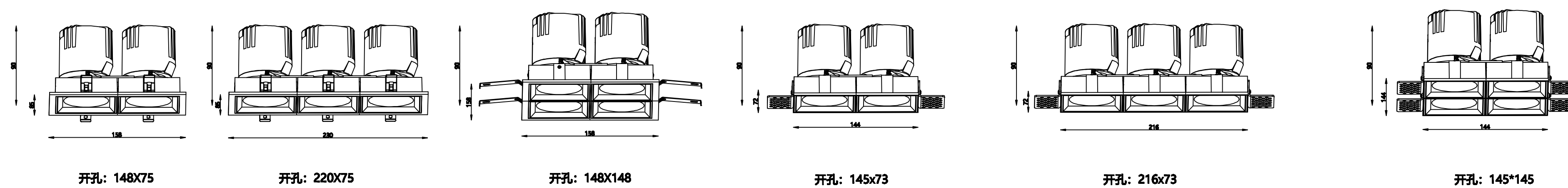
开孔: 148x75 开孔: 220x75 开孔: 148x148 开孔: 145x73 开孔: 216x73 开孔: 145x145
