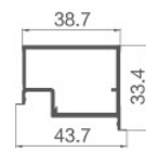
D-A635/ 龙骨 T: 1.4mm G: 0.583kg/m
