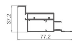
D-A632/ 主框 T: 1.4mm G: 1.102kg/m
