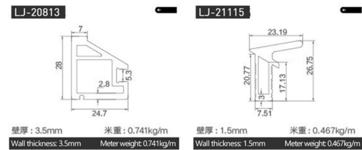
28 天地铰链框 28 air hinged frame
