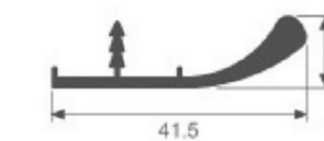
G-1325(BMW style)
