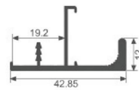
G-9229(Leather F Type Handle)
