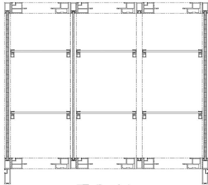
正面 (Front view)
