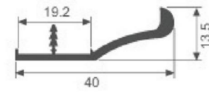
G-1324(M style)
