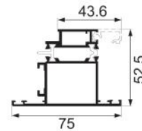
JNW-HC847A 75 new clip glass fan Weight : 1.45 kg/m
