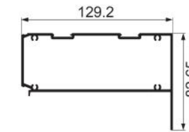
JNW-XT1185 intelligent top rail Weight : 2.26 kg/m
