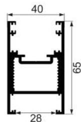
KY01-035 5.0-65 panels Weight : 1.72 kg/m
