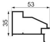
XY01-002F door casing Weight : 0.69 kg/m
