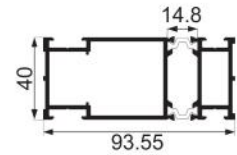
JNW-CT03-04 sash crossbar Weight : 2.07 kg/m
