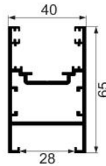
KY01-019 2.0-65 sashes Weight : 1.38 kg/m
