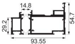
JNW-CT03-02 door panel Weight : 2.79 kg/m
