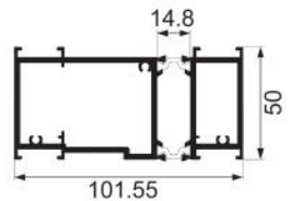
JNW-CT05-02 off-axis door upper frame Weight : 2.92 kg/m
