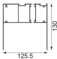
JNW-CT1584F 128 intelligent top rail Weight : 3.09 kg/m
