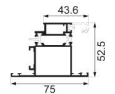
JNW-HC847A 75 new clip glass fan Weight : 1.45 kg/m
