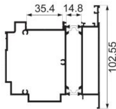
JNW-CT03-05 sash crossbar Weight : 2.63 kg/m
