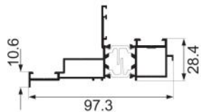
JNW-FK773A subframe Weight : 1.35 kg/m
