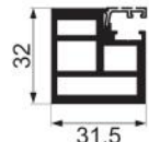
JNW-XT1465F hidden mesh door Weight : 1.26 kg/m
