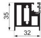
JNW-XT1464 mesh door bottom frame Weight : 1.36 kg/m
