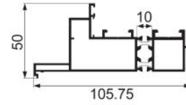
DZ-CT797F slim subframe Weight : 1.62 kg/m
