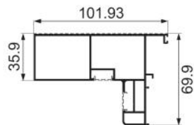
JNW-XT1470 handrail Weight : 1.58 kg/m
