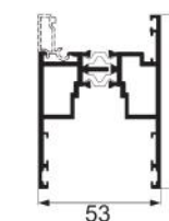
JNW-TS911F 75 lifting door Weight : 1.87 kg/m
