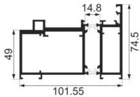
JNW-CT03-01 frame Weight : 3.51 kg/m
