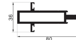
WB-80002 Name : 80 center column Weight : 1.558 kg/m
