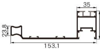
JY-WP-83 Name : handle Weight : 1.78 kg/m
