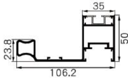
JY-WP-98 Name : handle Weight : 1.47 kg/m
