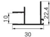
OPK-A329 Name : frames Thickness : 1.0mm Weight : 0.24 kg/m
